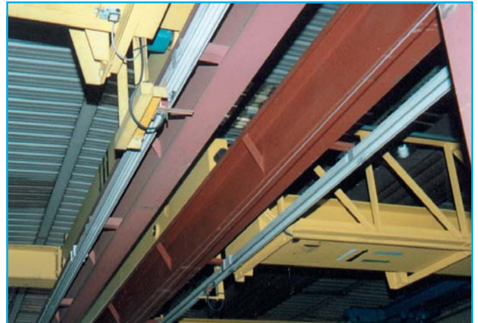
Fig. 2 - Principe d'entraînement et de raccordement électrique du chariot-collecteur sur pont roulant posé (voir fig. 4).
