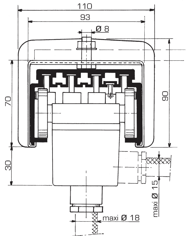
Fig. 1 - Coupe de la POLYGAINÉ avec encombrement pour : - chariot-collecteur MA 432 - griffe de suspension CP 506 - éclisse jumelée CP 504
